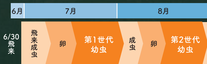
■図1／飛来時期に基づくトビイロウンカの発生予想パターン図の例
